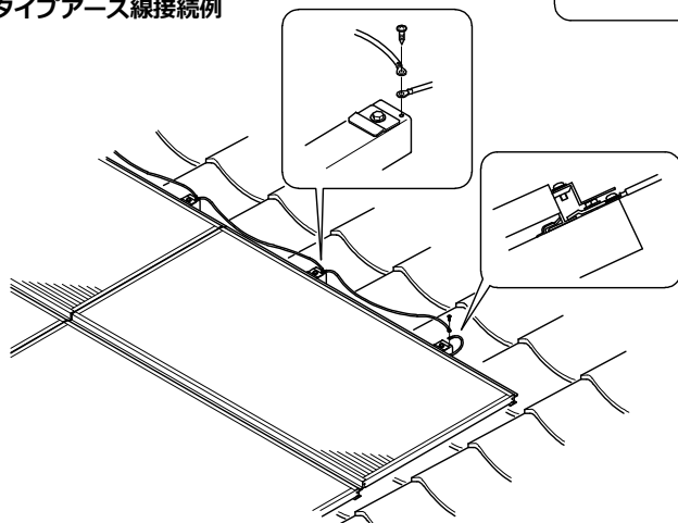
傾斜屋根タイプアース線接続例
