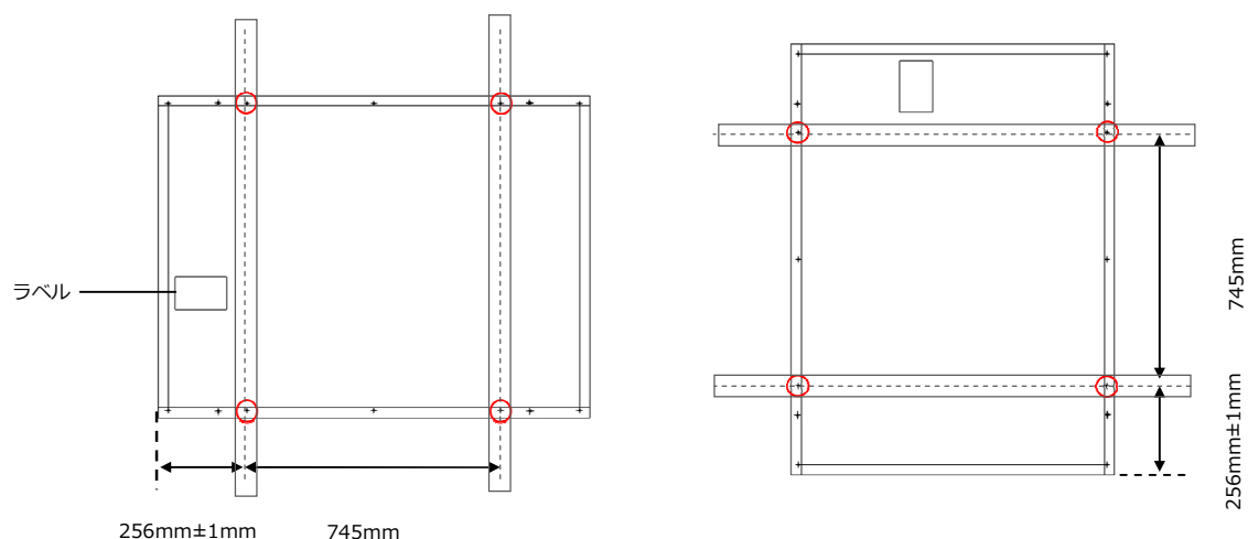
モジュール裏面図
