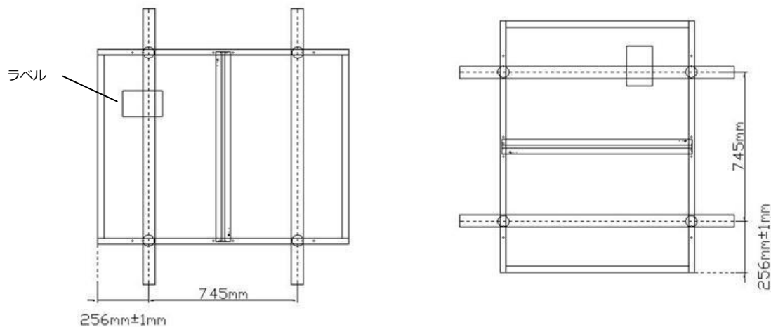
太陽電池モジュール裏面図
