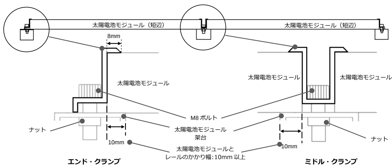
アレイ設置(断面図)
