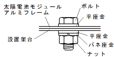
拡大部
