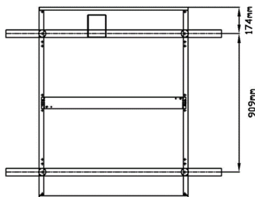
縦向き設置
