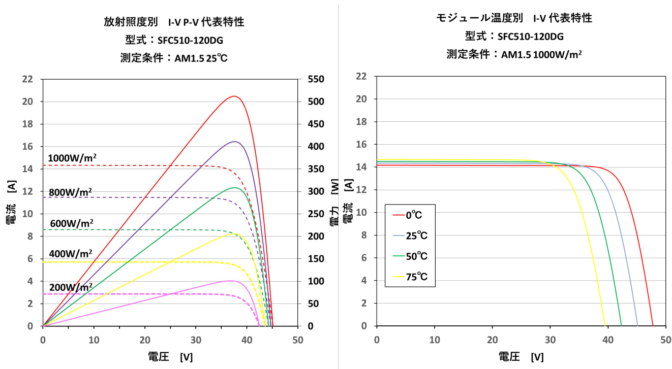
図 10 代表的な照度、温度特性
